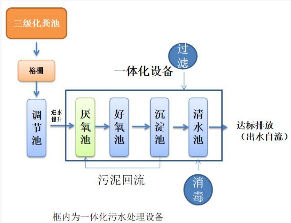
图3-3 污水处理工艺图
