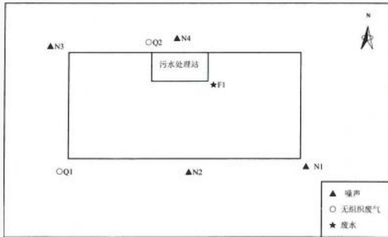
图7-1 验收监测布点图
