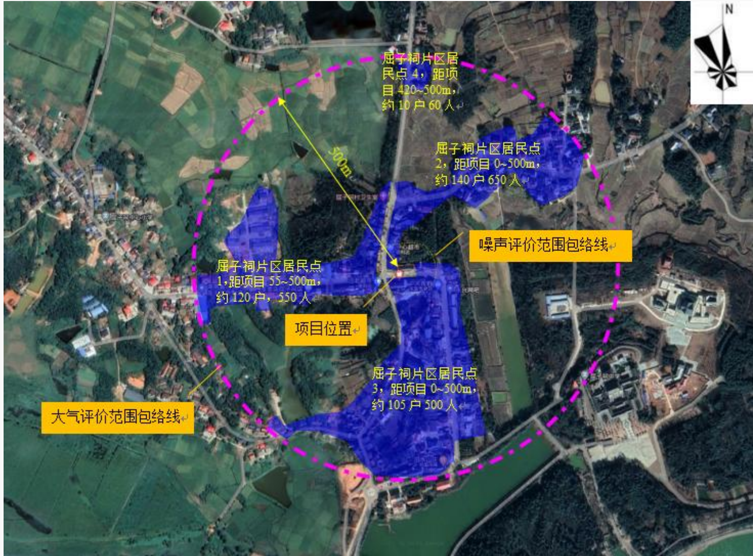
附图3 项目周边环境现状及环境保护目标示意图
